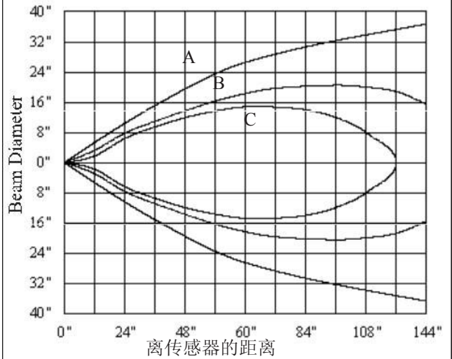
典型的RPS-409A-144/216-IS2波束图形
