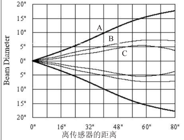
典型的RPS-409A-144/216-IS2波束图形
